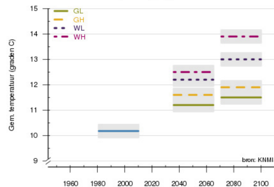
Langjarig gemiddelde jaartemperatuur voor De Bilt in het verleden (blauw) en voor de KNMI'14 scenario's met natuurlijke variabiliteit tussen 30-jaar perioden (grijs)
